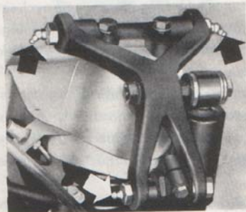
Bild 32. Övre länkmarm.
