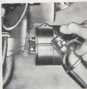
Bild 31. Generator (B 16 A, B 18 A).
