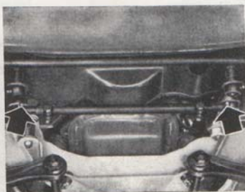
Bild 36. Parallellstagg. Beträffande kulleleder utan smörjnipp- lar, se sid. 7.
