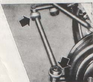
Bild 35. Styrstag. Beträffande kulleleder utan smörjnipp- lar, se sid. 7.
