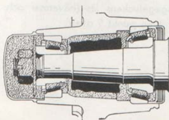
Bild 26. Framhjulslager.
