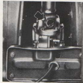
Bild 39. Främre kardanknut.
