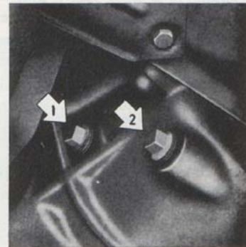
Bild 3. Växellåda. 1. Påfyllningspropp 2. Avtappningspropp
