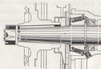
Bild 27. Bakhjulslager.
