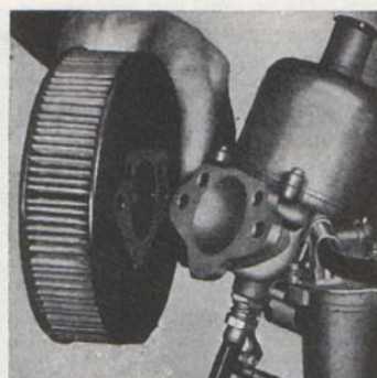
Bild 16. Byte av luftrenare (B 16 B, B 18 D).
