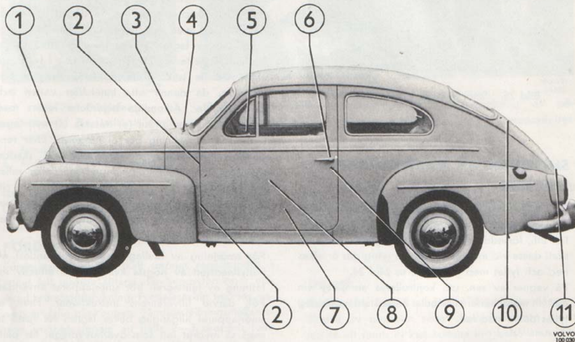
Bild 28. Smörjställen på kaross, PV 544.
