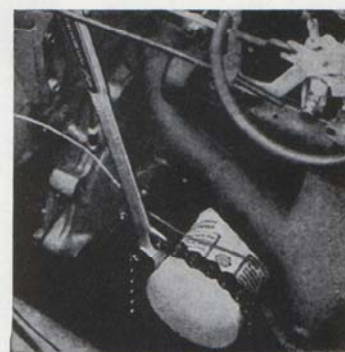
Bild 9. Demontering av oljerenare (B 18).
