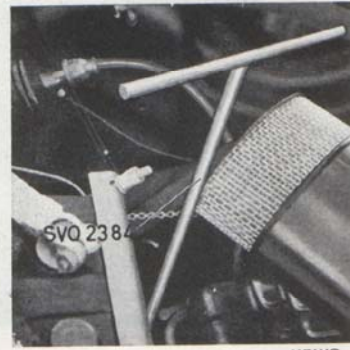
Bild 22. Demontering av påfyllningspropp i huvudcylinder.
