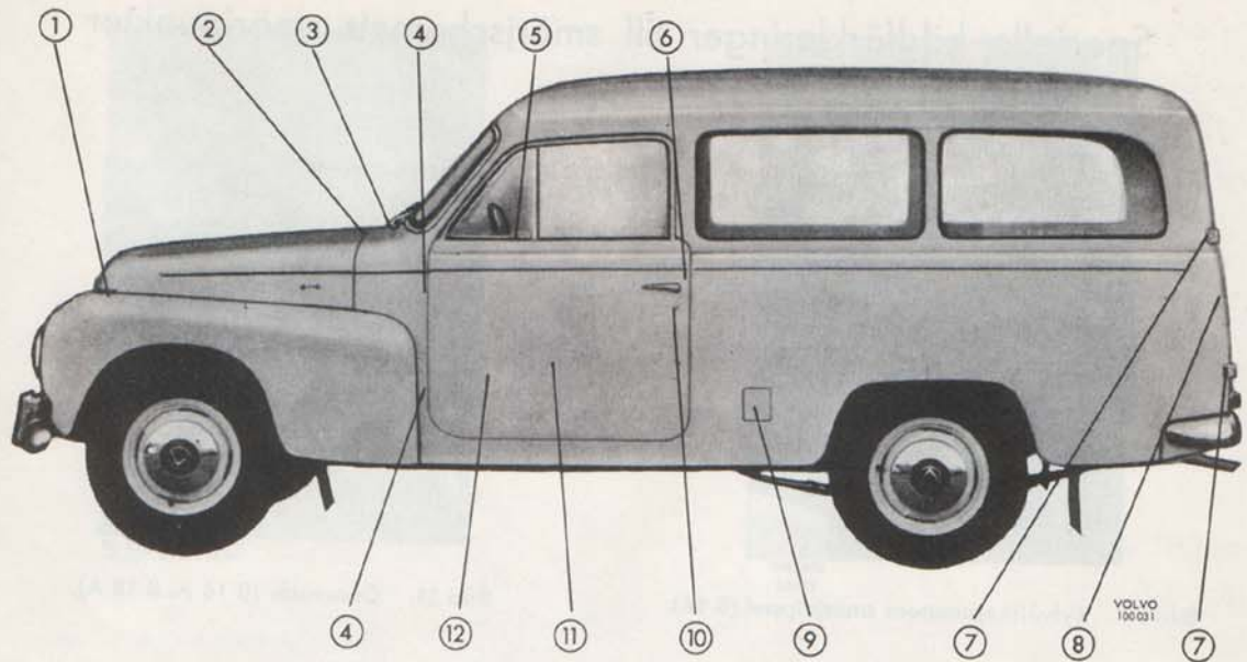
Bild 29. Smörjställen på kaross, P 120.
