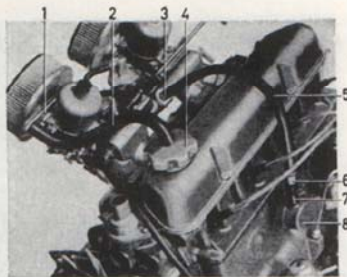
Bild 11. Positiv vevhusventilation.
