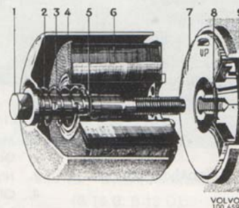
Bild 8. Smörjoljerenare (B 16).
